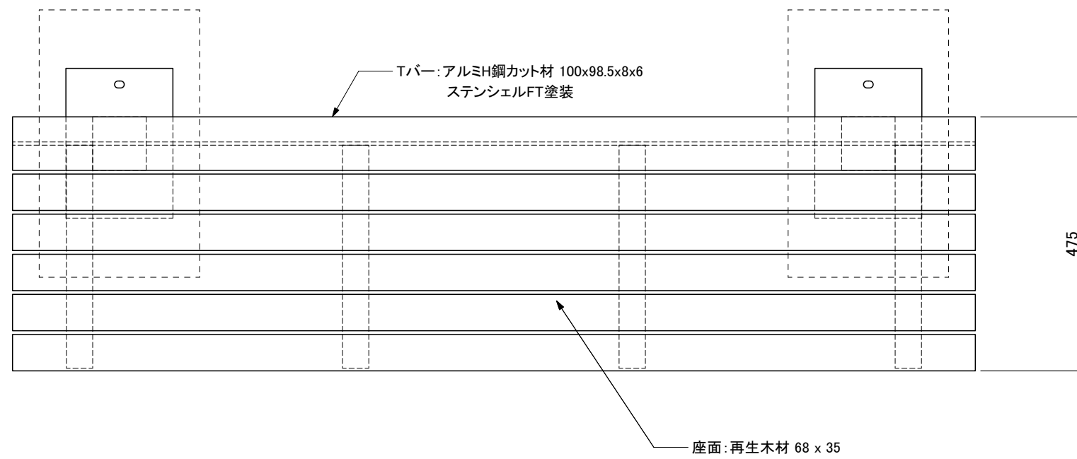
平面図
