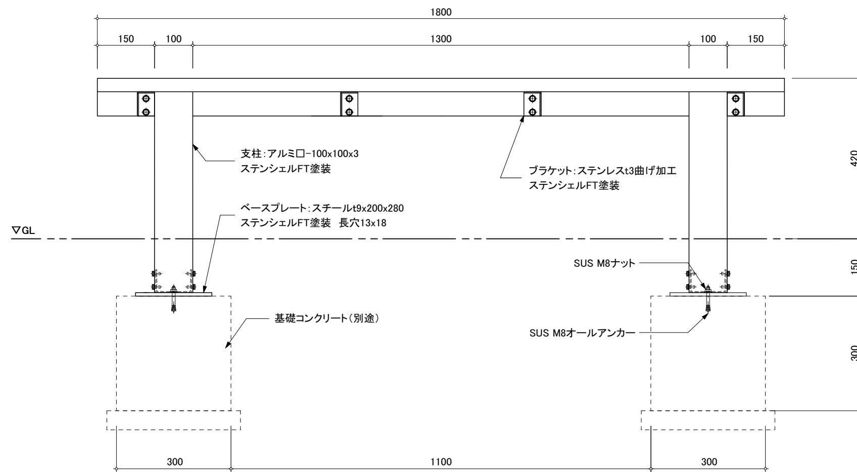
正面図
