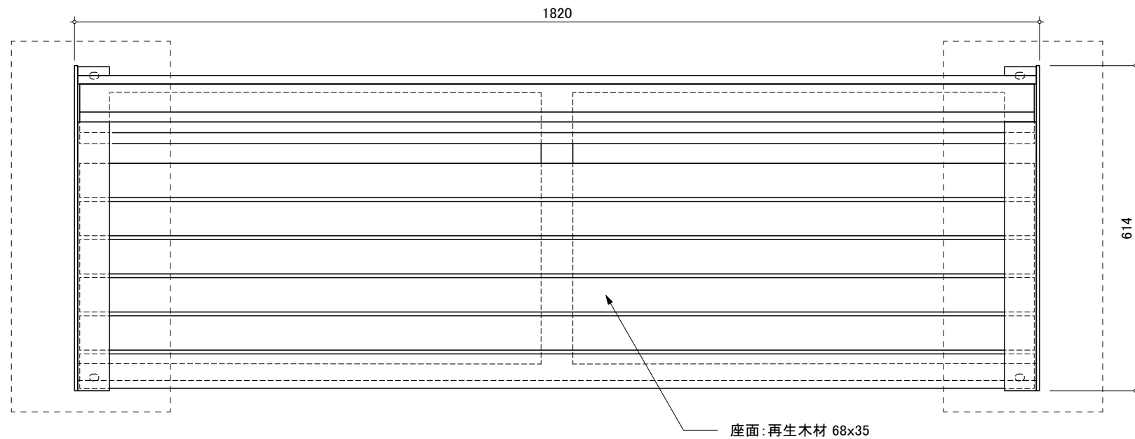
平面図
