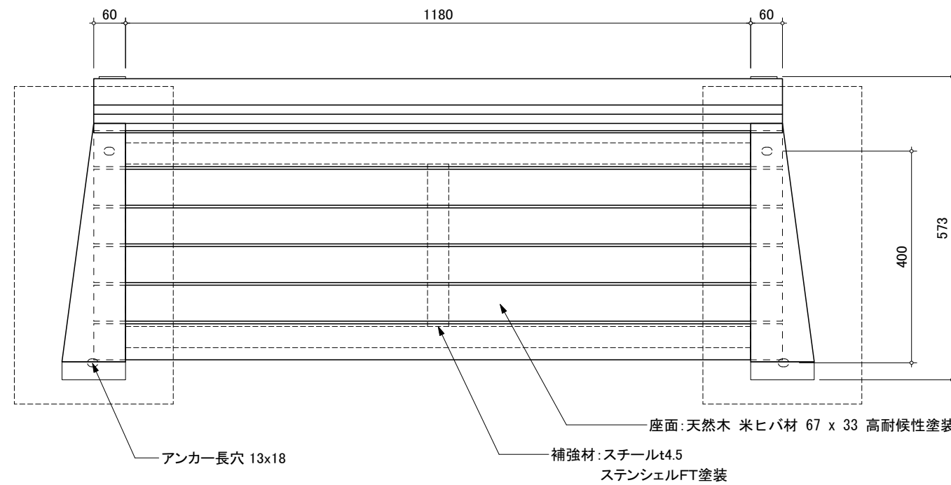
平面図
