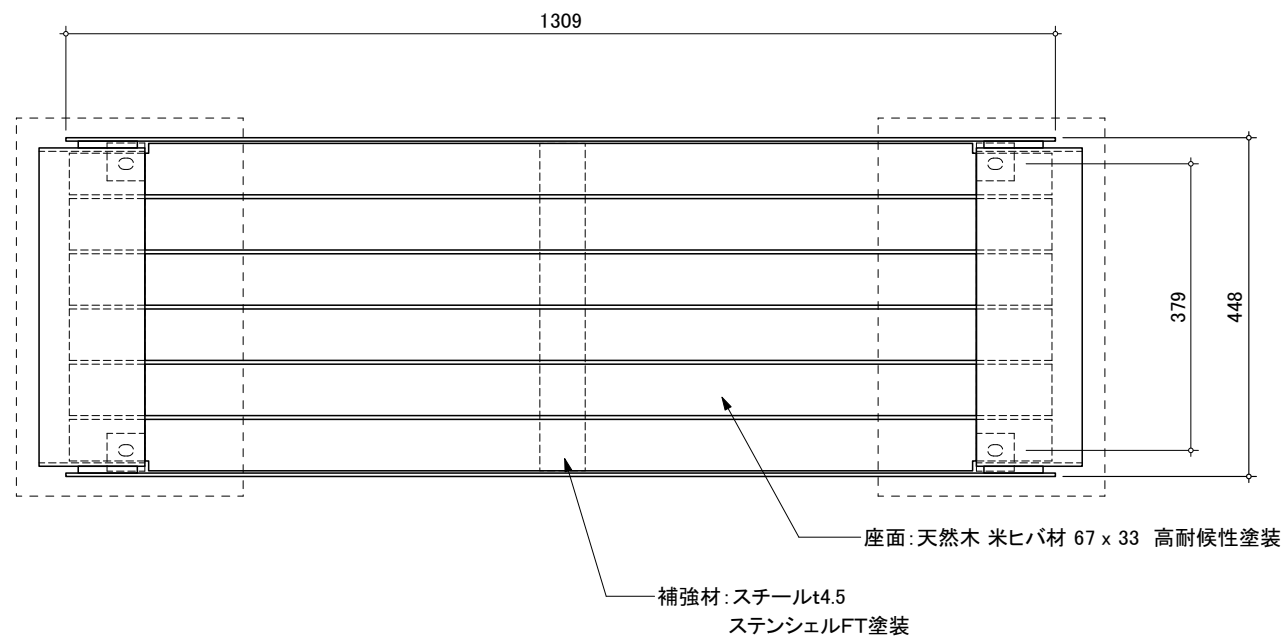
平面図
