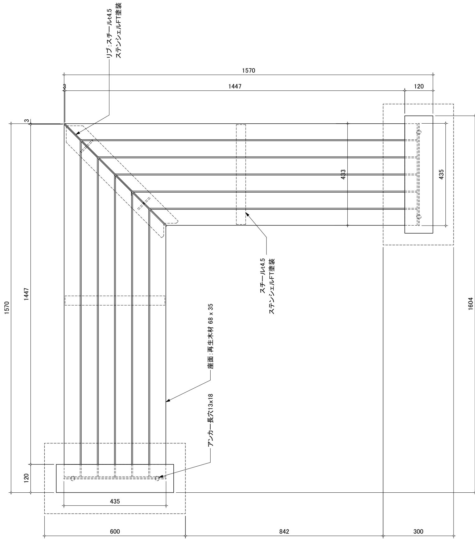
平面図
