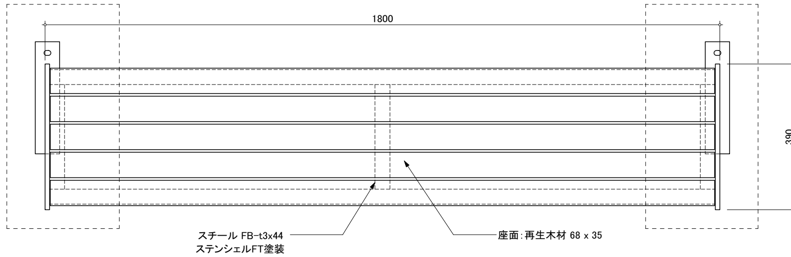
平面図
