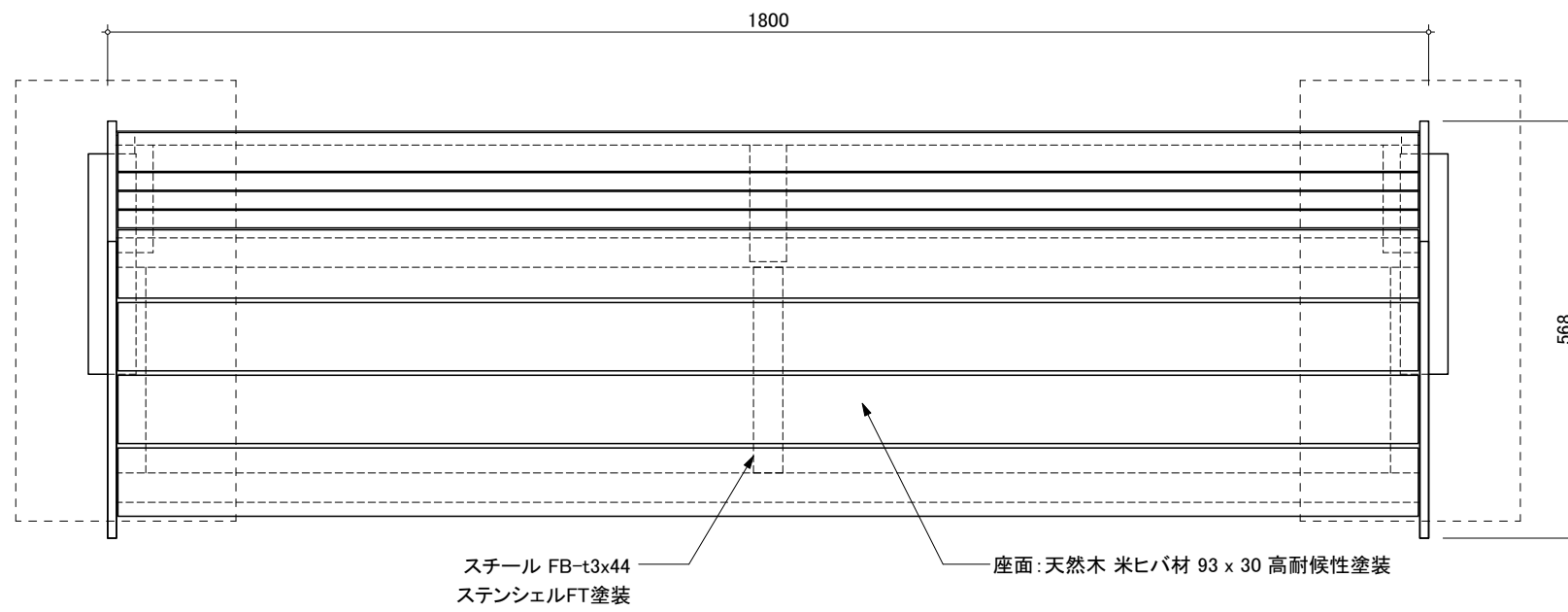
平面図
