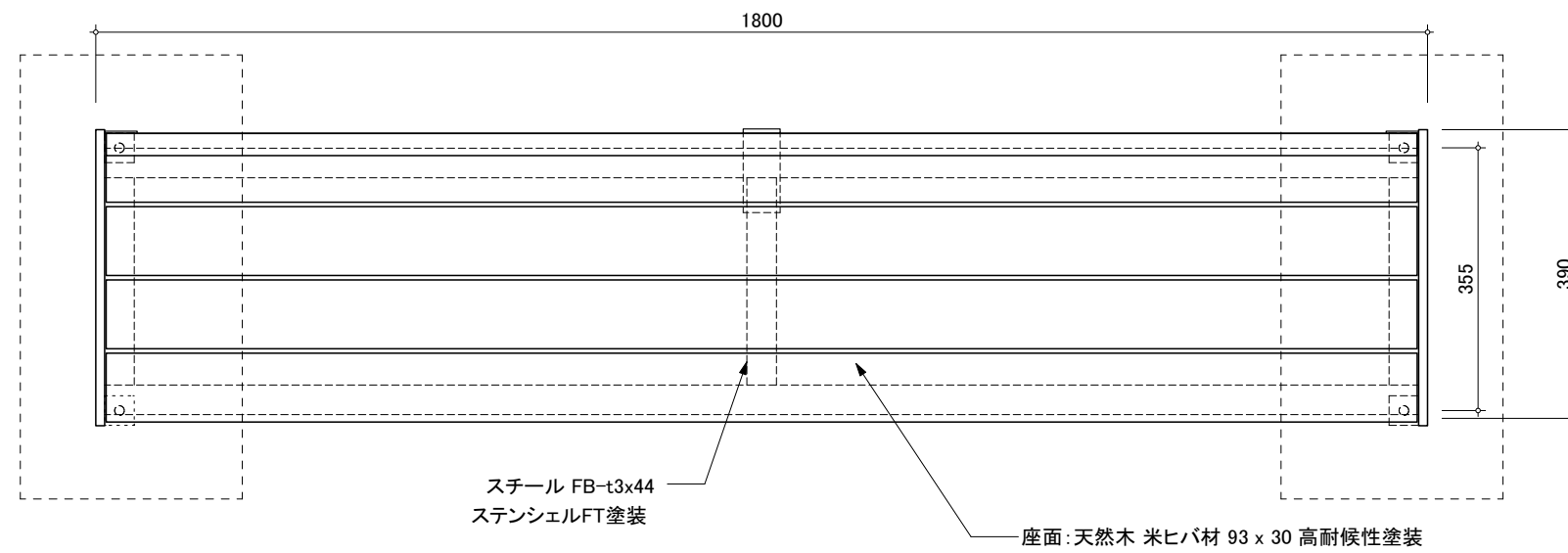
平面図
