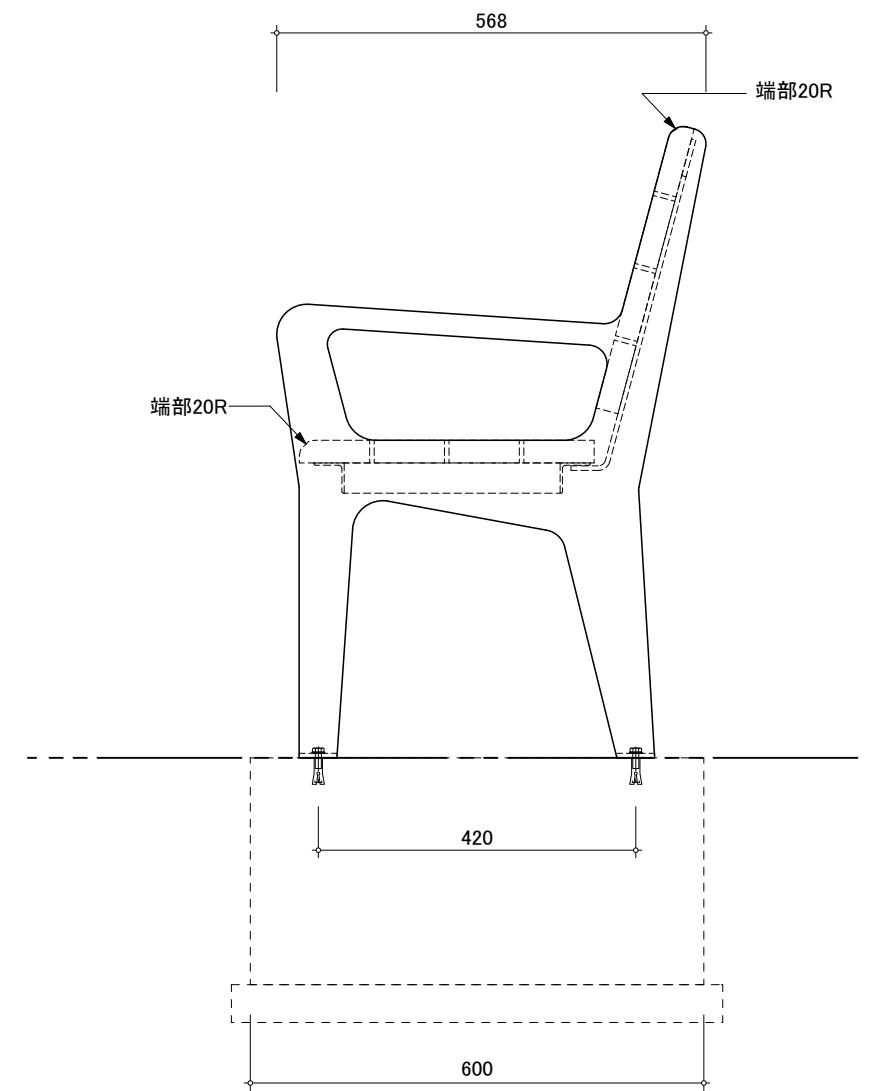
側面図
