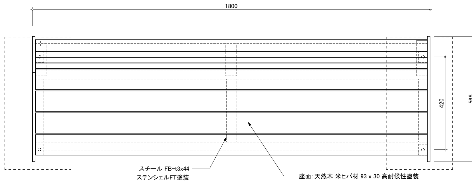
平面図
