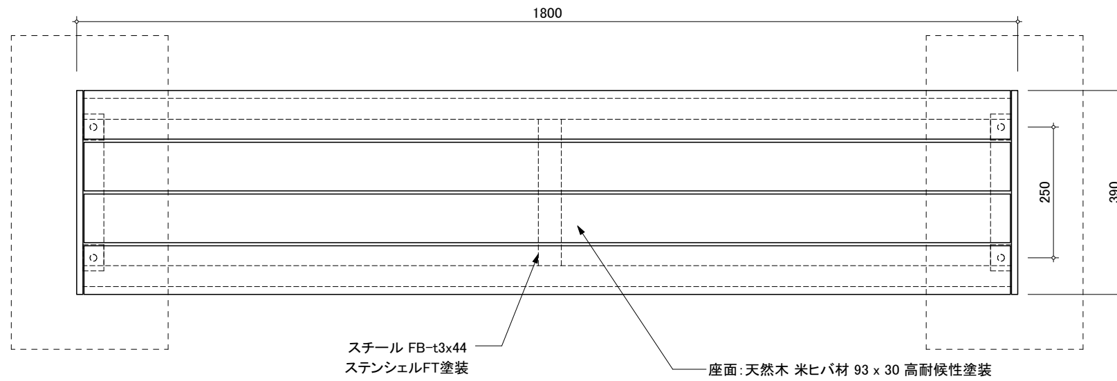
平面図
